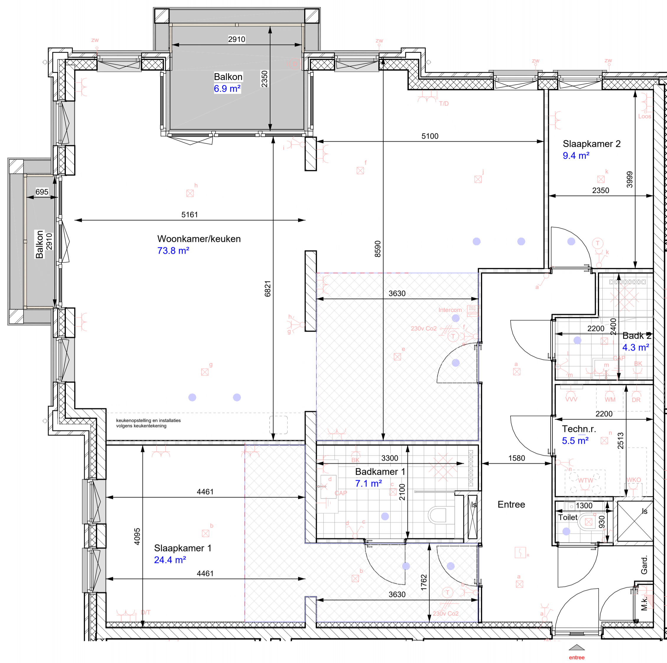
Plattegrond
